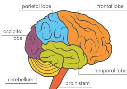
Figura 8- Lobos Cerebrais.
