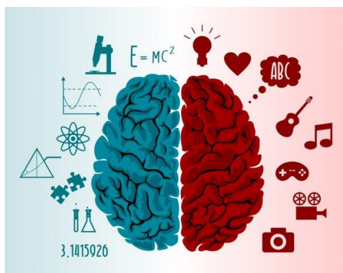
Figura 9- Hemisférios cerebrais.
